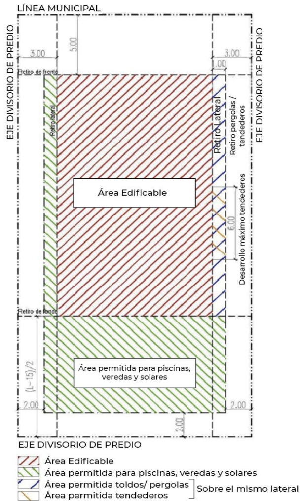
Esquema de retiros de lote típico
