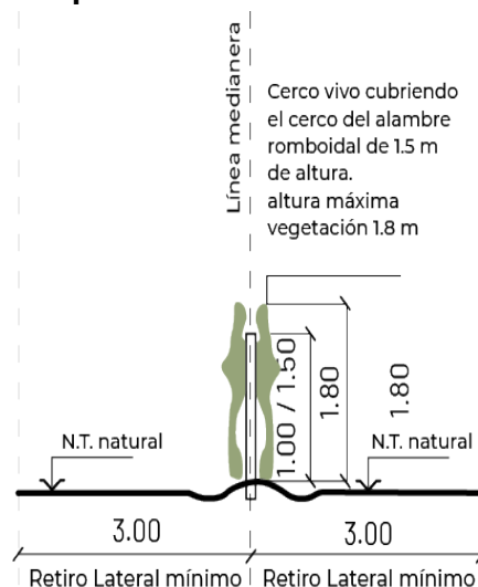
Esquema de cerco medianero
